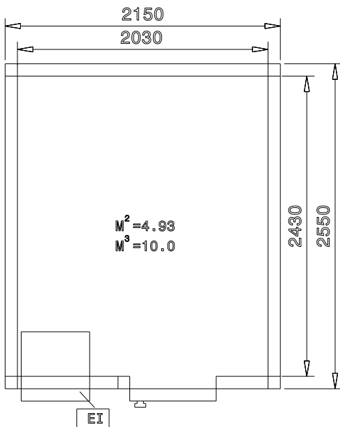
Boven aanzicht
