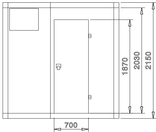
Zij aanzicht
